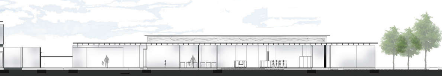
Corte Longitudinal
