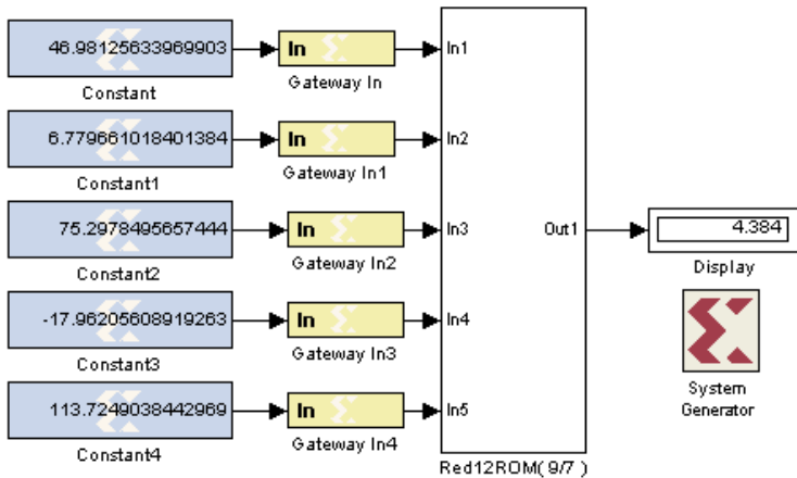
Figura 6: Red neuronal para estimación de resistencia rotórica.
