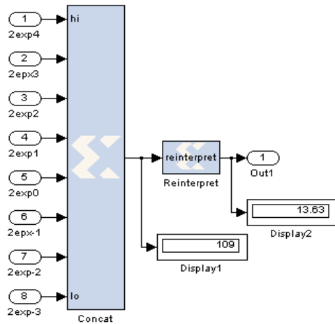
Figura 8: Bloque para la conversión análogo-digital.
