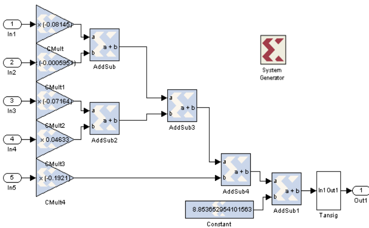
Figura 5: Modelo en Sysgen de una neurona estándar.
