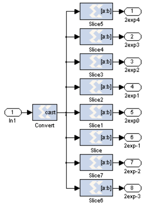
Figura 7: Bloques para la conversión digital-análoga.
