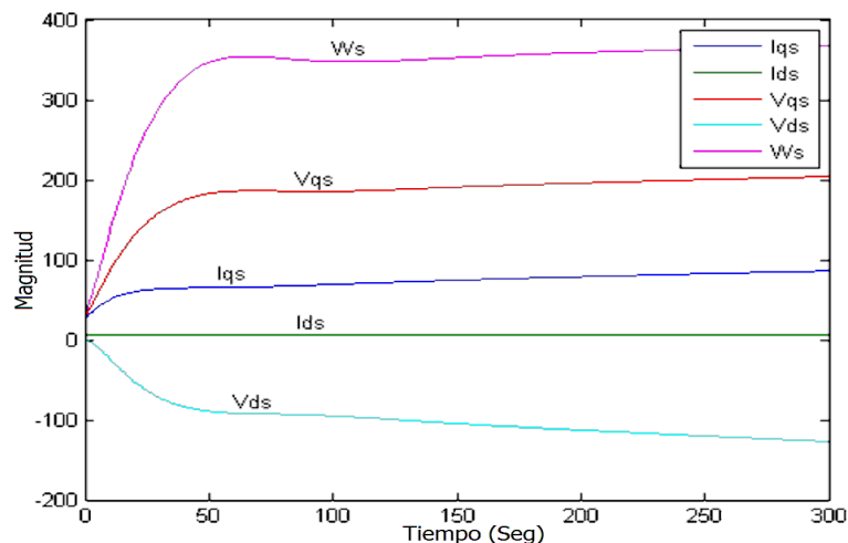
Figura 4: Gráfica del comportamiento de las entradas de la red neuronal.
