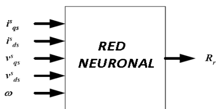
Figura 3: Red neuronal para estimación de resistencia rotórica.
