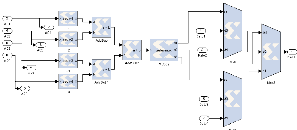
Figura 12: Bloque de selección de dato.
