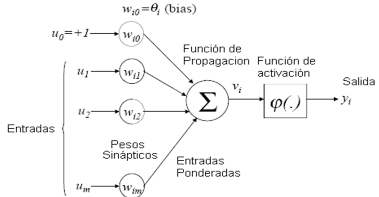
Figura 1: Modelo de una neurona artificial.
