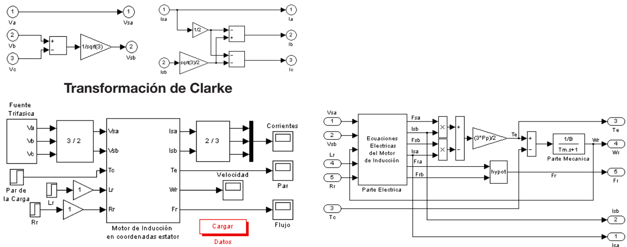
Figura 2: Modelo del MI. a) Diagrama en Bloques. b) Modelo del motor.
