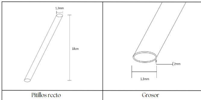
Figura 3. Plano técnico del pitillo Fuente: Propia.
