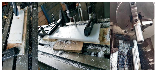
Figura 4. Mecanizado de chasis, Fuente: Autor
