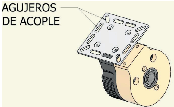
Figura 2. Modelado de acople para herramientas, Fuente: Autor
