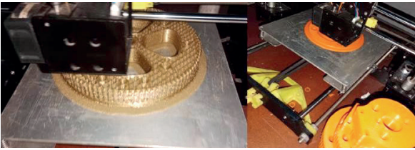
Figura 5. Impresión de piezas impresas en 3D, Fuente: Autor En la figura 6 se pueden observar todas las piezas de impresión 3D ya fabricadas junto a las piezas mecanizadas mediante procesos de torneado y fresado.
