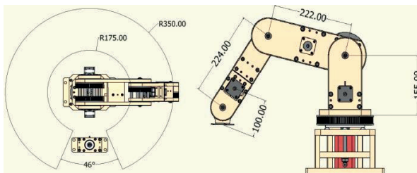
Figura 3. Dimensiones generales del diseño, Fuente: Autor
