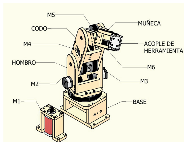
Figura 1. Diseño CAD del brazo, Fuente: Autor
