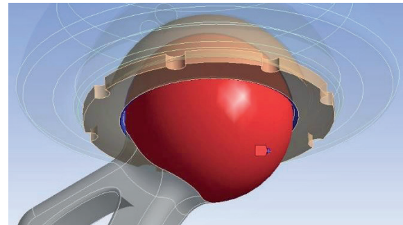
Figura 4. Contacto no lineal entre la esfera femoral y el componente medioacetabular.
