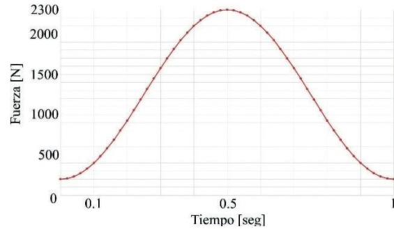
Figura 7. Gráfica de la carga aplicada.
