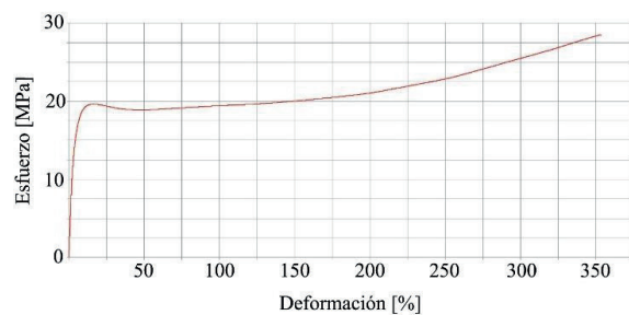
Figura 3. Gráfica esfuerzo-deformación real del UHMWPE.
