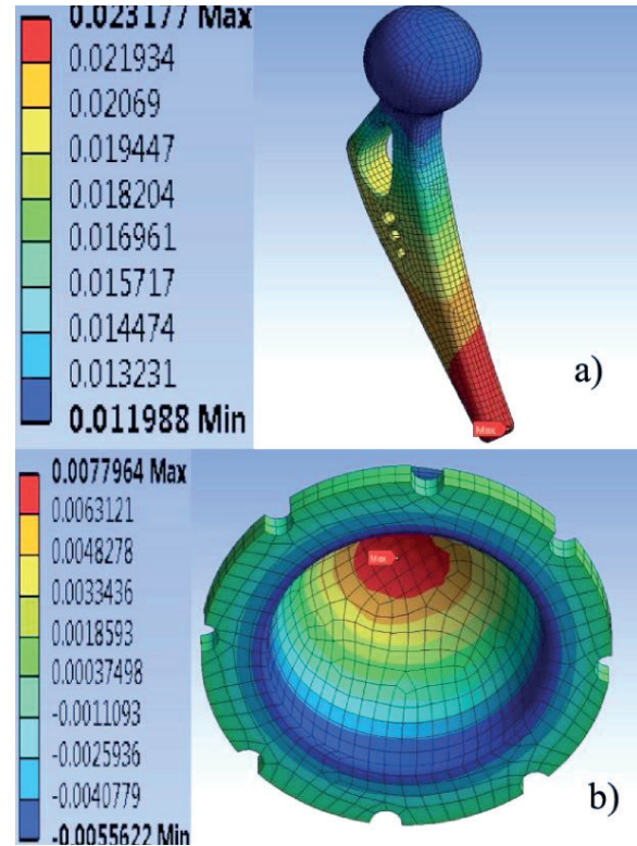
Figura 9. a) Desplazamientos en la hemiprótesis, b) desplazamientos en componente acetabular medio. Todas las unidades en mm.
