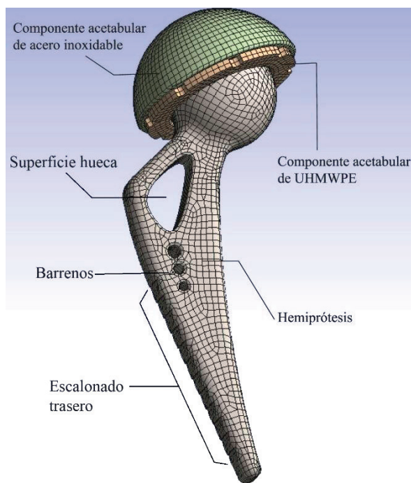
Figura 2. Modelo de la prótesis total de cadera.
