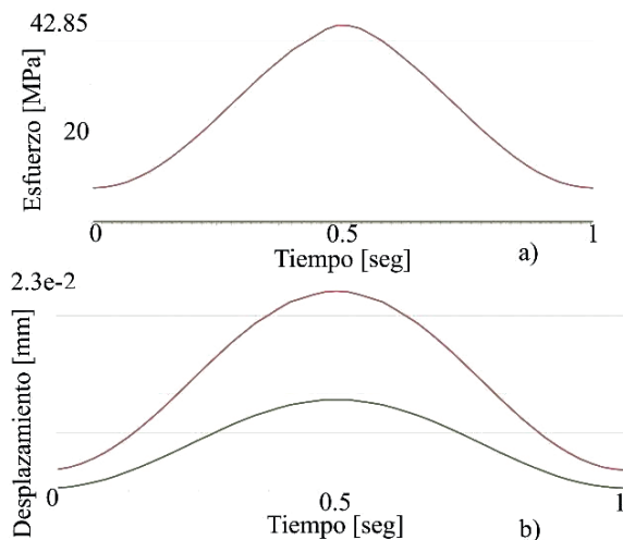
Figura 10. a) Gráfica del comportamiento de los esfuerzos en la hemiprótésis, b) Gráfica de los desplazamientos equivalentes en la hemiprótésis.
