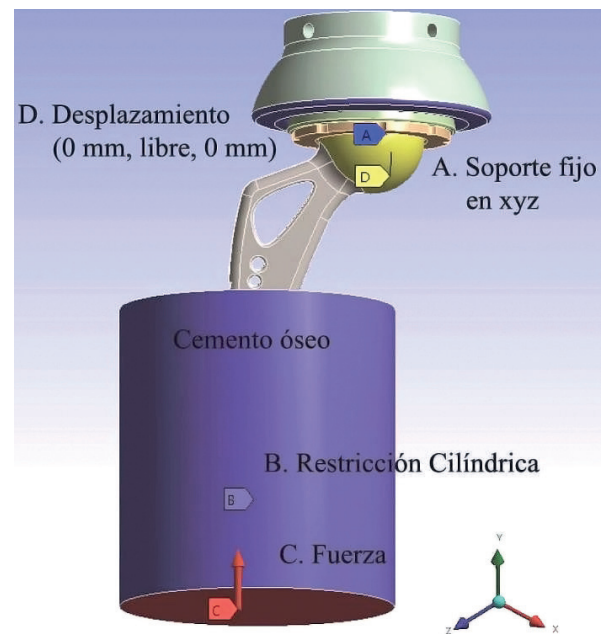
Figura 5. Condiciones de frontera generales.
