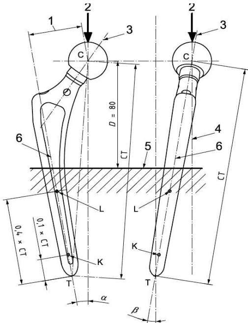
Figura 6. Posicionamiento de la prótesis para la prueba.
